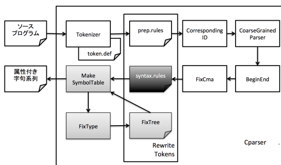
図 9 拡張後の TEBA の全体像
